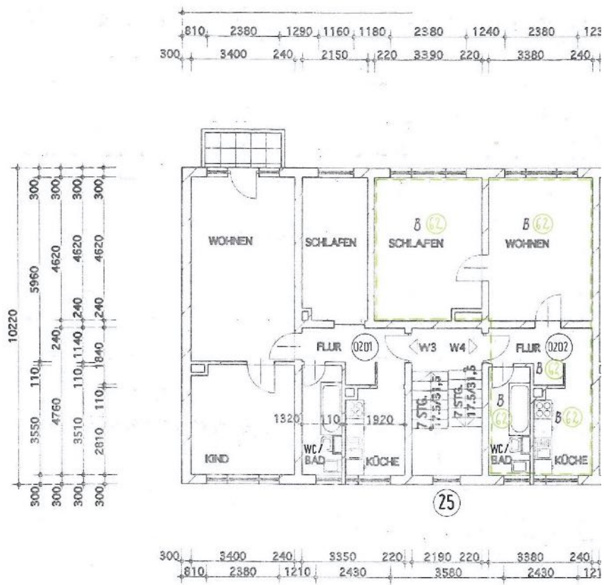
1.OG Grundriss
